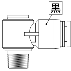
ワンタッチ管継手 ELB075
